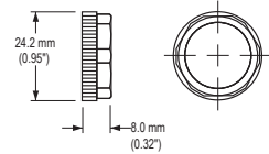
Figura 6. Dado di bloccaggio
