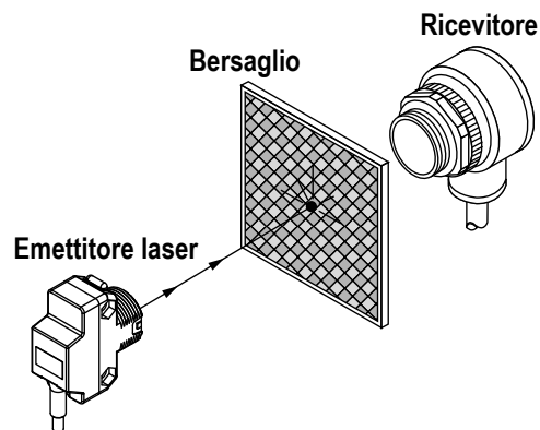
Figura 2. Allineamento a lunghe distanze
