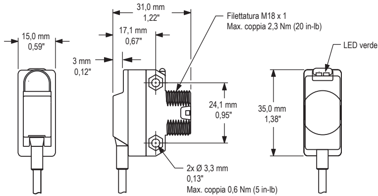
Figura 4. Modelli con cavo integrato
