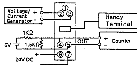
Fig. 9: Wiring Diagram
