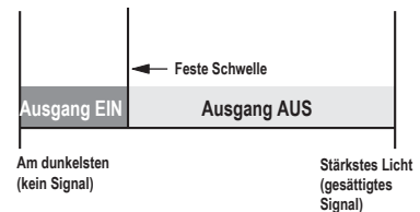
Abbildung 3. Erfassungsbetriebsart DARK SET in Dunkelschaltung
