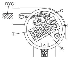
Remote type detector (DY-N.../E1)
